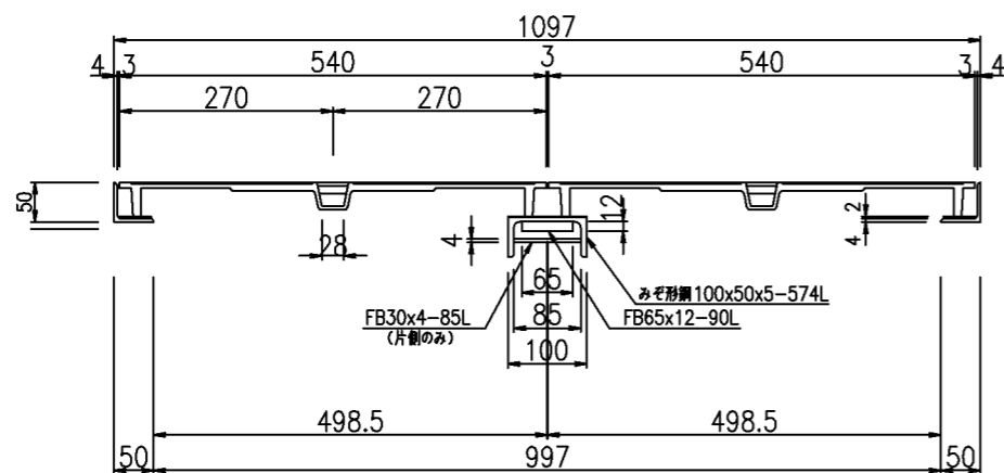
C-C断面図
