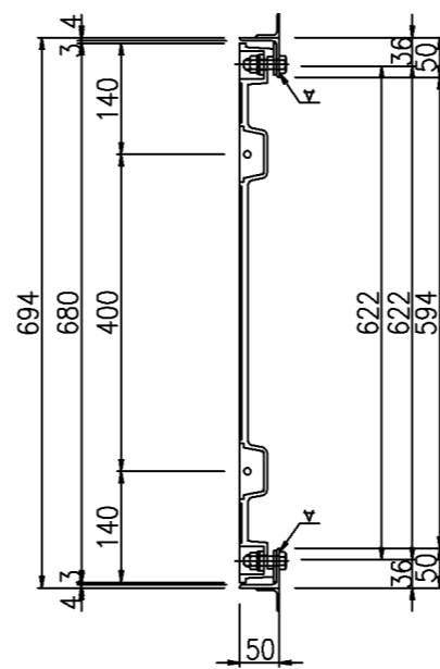
A-A断面図
