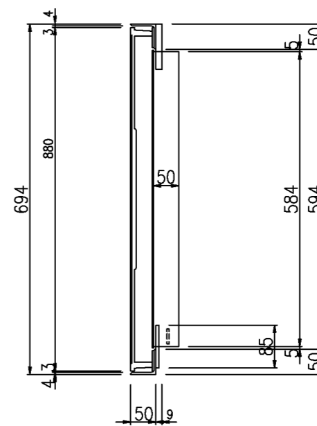
B-B断面図
